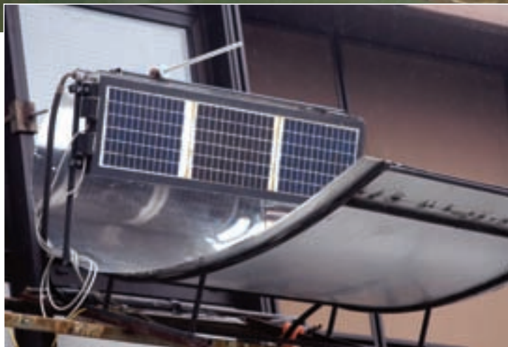
КОЛЕКТОР ЗА СОЛАРНУ ЕНЕРГИЈУ
