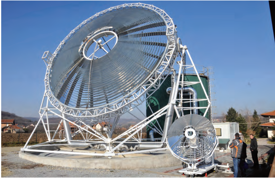
ПОСТРОЈЕЊЕ КОЈЕ САКУПЉА СУНЧЕВУ ЕНЕРГИЈУ
