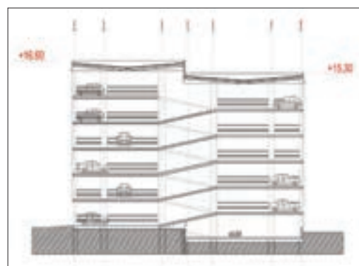
ПРЕСЕК КОЈИ ПОКАЗУЈЕ СПРАТНОСТ
